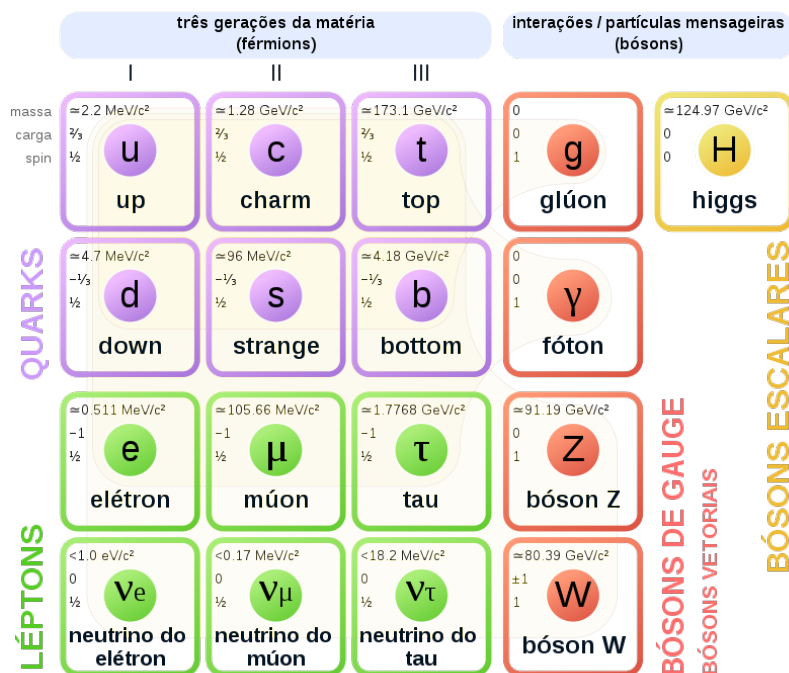
Figura 4.2: Modelo Padrão de Partículas Elementares.
