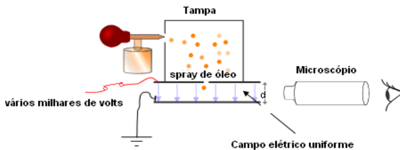
Figura 5.6: Representação do aparato experimental de Millikan.
