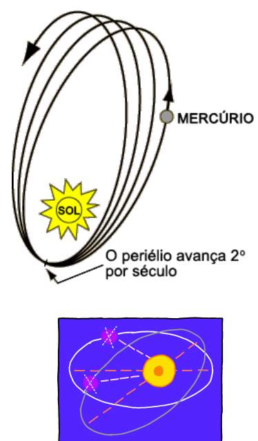
Figura 1.9: Precessão do periélio de Mercúrio: a Mecânica Newtoniana prevê que o periélio (ponto mais próximo do Sol) da órbita de um planeta é alterado com o tempo; porém havia uma diferença entre o valor esperado e o valor medido para a órbita de Mercúrio, que só foi solucionada com a Mecânica Relativística.
