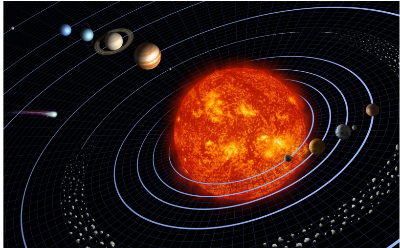
Figura 3.8: Imagem ilustrativa do sistema solar. Fonte: Harman Smith and Laura Generosa, Wikimédia Commons.
