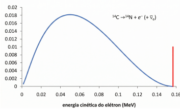
Figura 5.27: Energia esperada do elétron emitido no decaimento beta (vermelho) e o espectro de energia observado para o elétron (azul).
