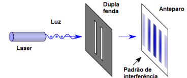
Figura 5.16: Padrão de interferência formado pelo experimento de dupla fenda.
