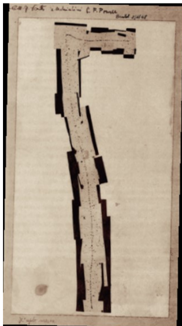
Figura 7.3: Decaimento Méson-Pi em Múon. (Assinado por: César Lattes, Cecil Powell e Giuseppe Occhialini)
