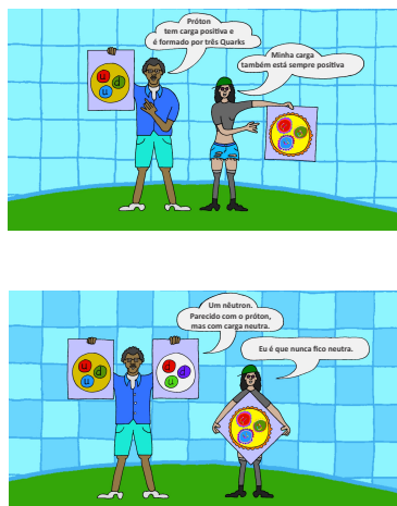
Figura 5.23: Representação de um próton. Não existe uma forma de enxergarmos um próton, então a criatividade é o limite. Ele tem carga positiva e é formado por três quarks de valência: (uud). Já o nêutron é parecido com o próton mas com carga elétrica neutra e formado por três quarks também: (udd).
