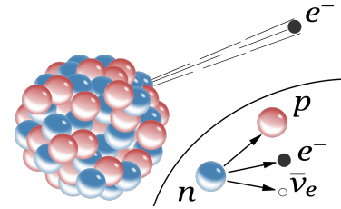
Figura 5.24: Decaimento Beta. Fonte: Inductiveload, Wikimedia Commons.
