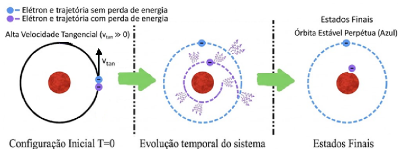
Figura 3.16: Um elétron clássico perderia energia devido a emissão de radiação ao ser acelerado. Porém, Bohr postula que existem órbitas estáveis onde isto não acontece e o elétron pode manter trajetórias elípticas.
