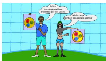
Figura 3.17: Um próton é formado por três quarks e tem carga positiva.
